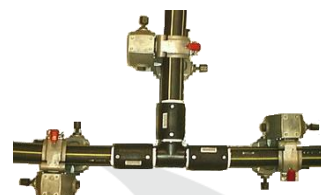
Té
